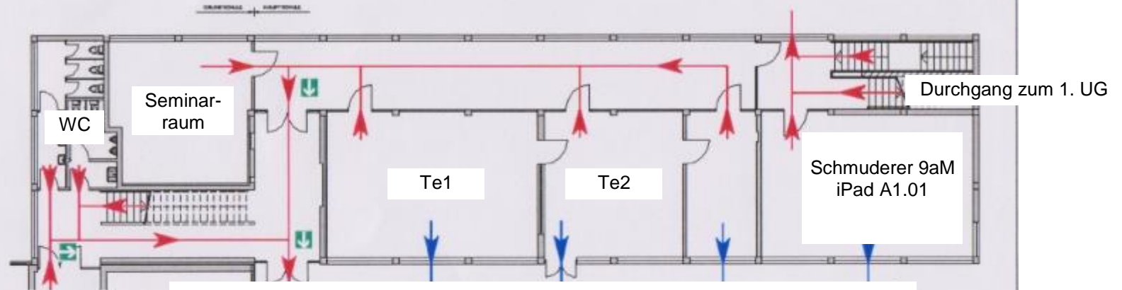
Anbau Mittelschule – EG
